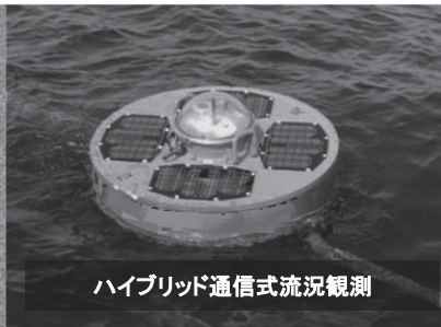
長期海流観測用漂流ブイ
