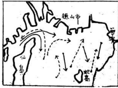
オ2図 徳山湾の潮流。 —————> 下ダ潮。 - - - - -> 上ダ潮。
